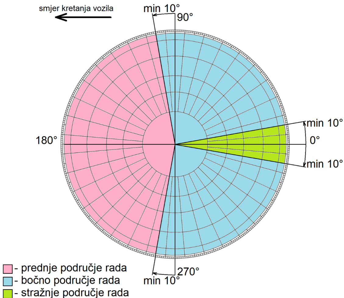
Dijagram radnih područja kрана
