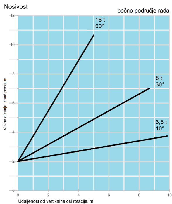
Dijagram nosivosti bočnog područja rada
