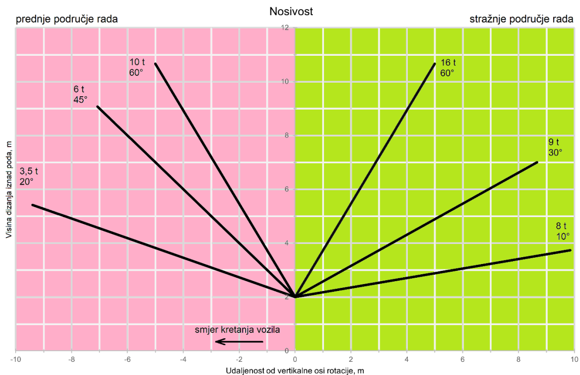
Dijagram nosivosti prednjeg i stražnjeg područja rada
